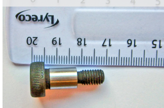
Ansattsskruv för gummirep Shoulder Screw for Rope
